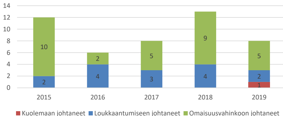
Tieliikenneonnettomuudet Reisjärvellä 2015-2019
